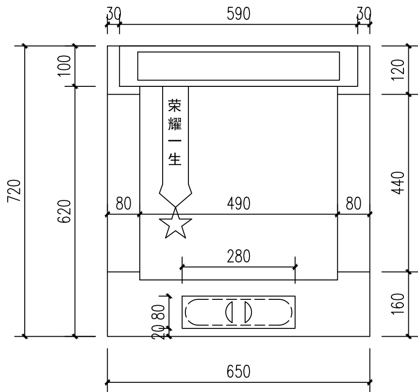
平面图
