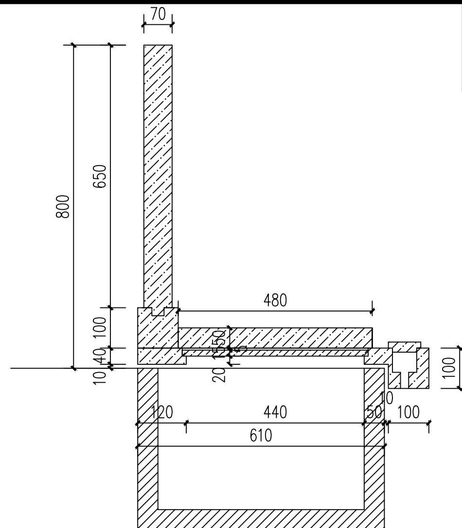
剖面图
