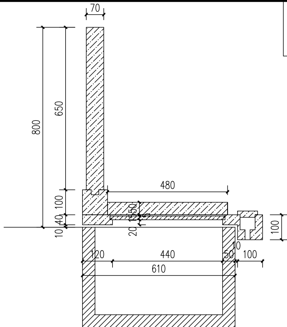
剖面图
