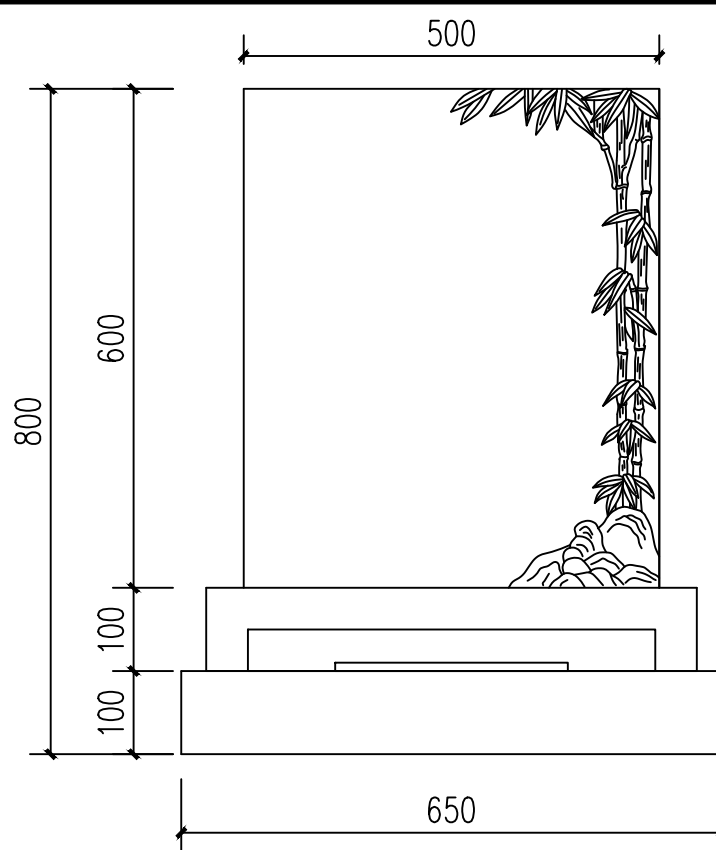
立面图
