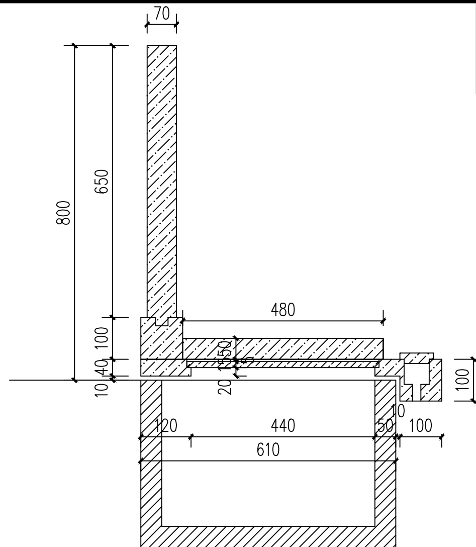
剖面图
