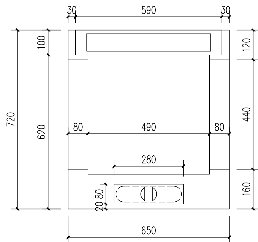
平面图
