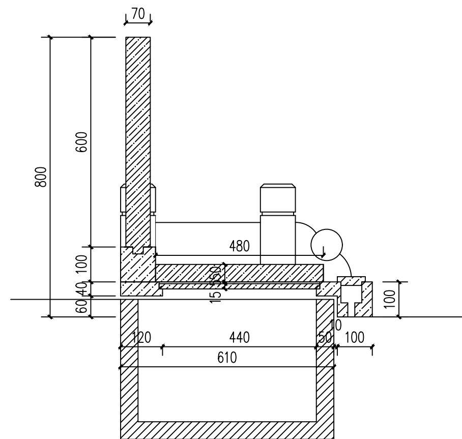
剖面图
