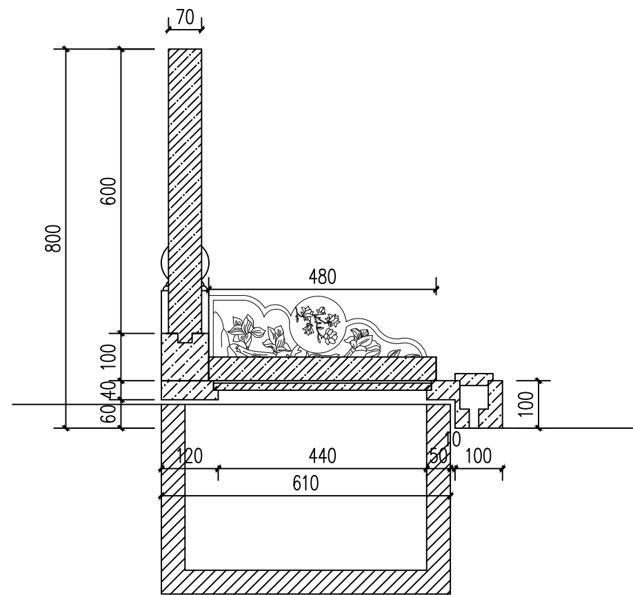
剖面图
