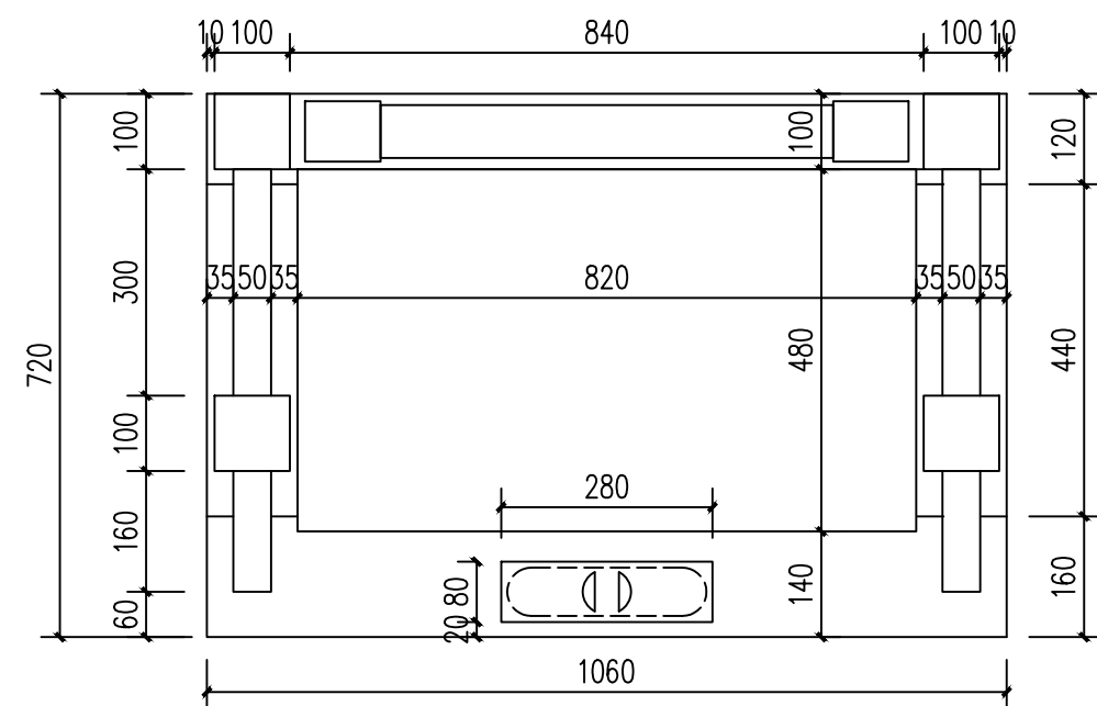
平面图
