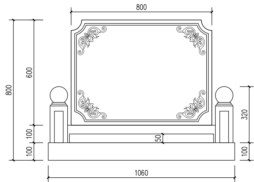
立面图
