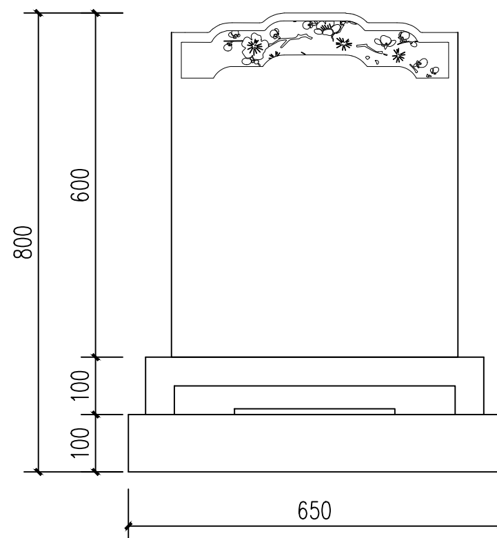
立面图
