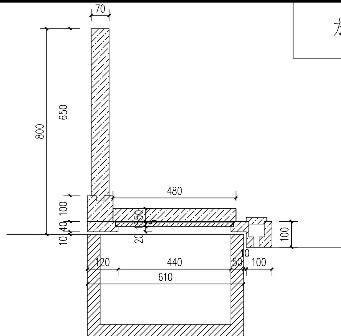
剖面图
