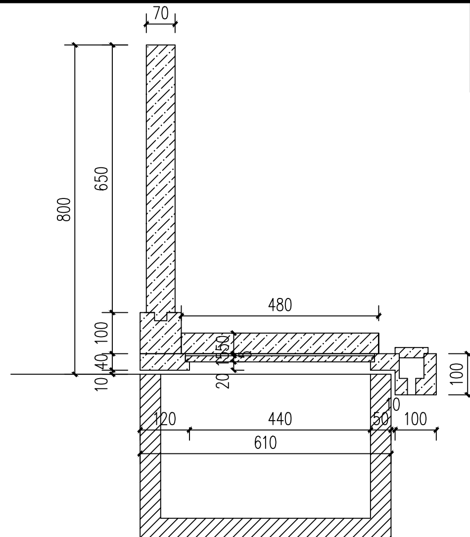
剖面图
