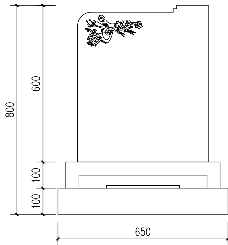
立面图
