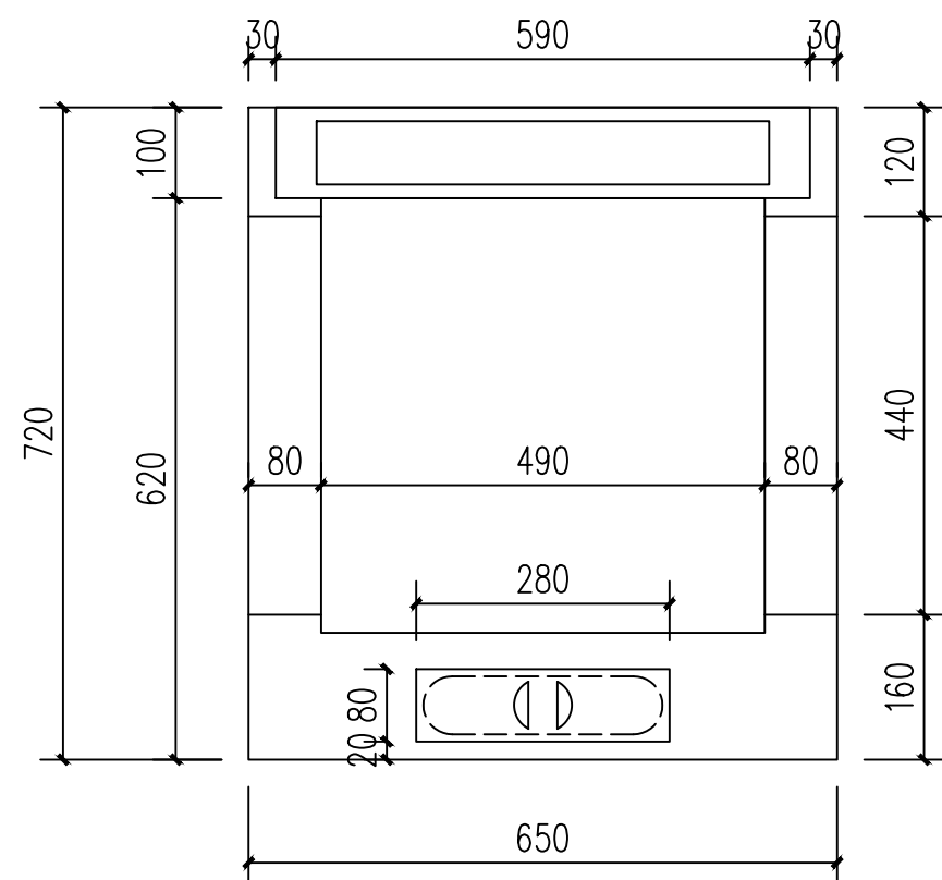
平面图
