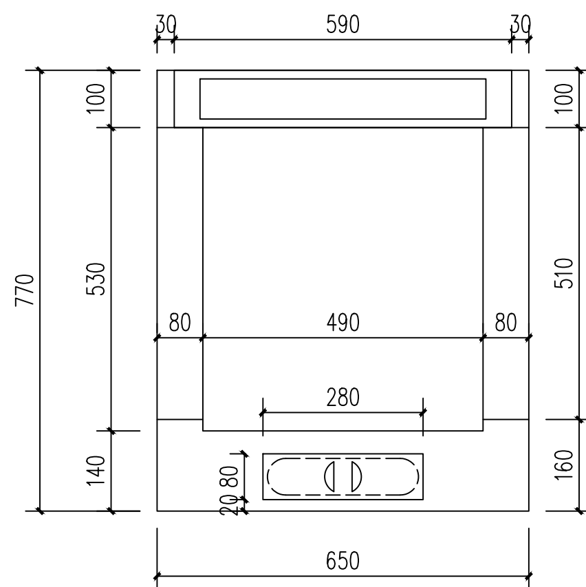
平面图
