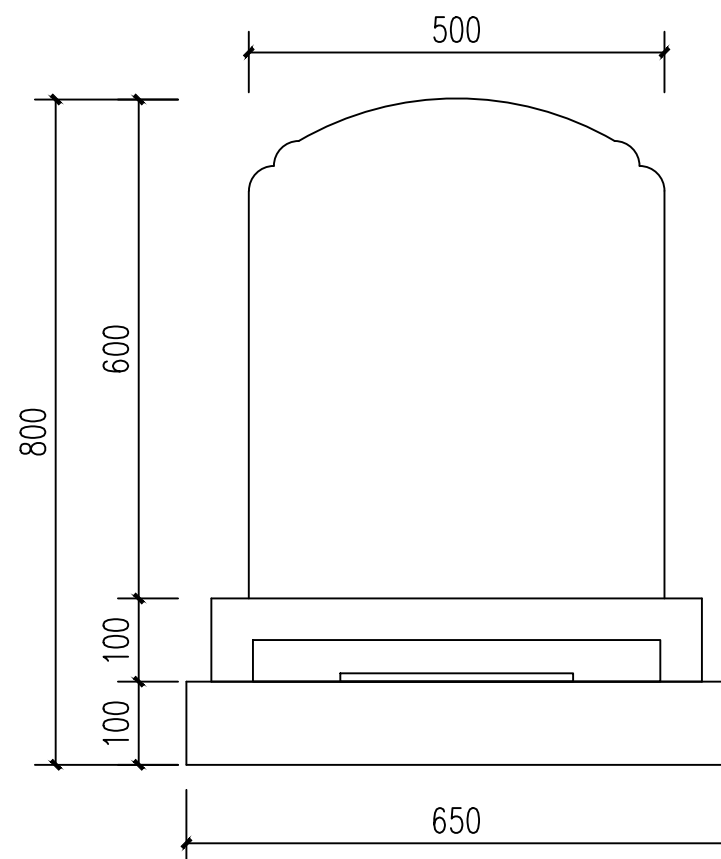
立面图
