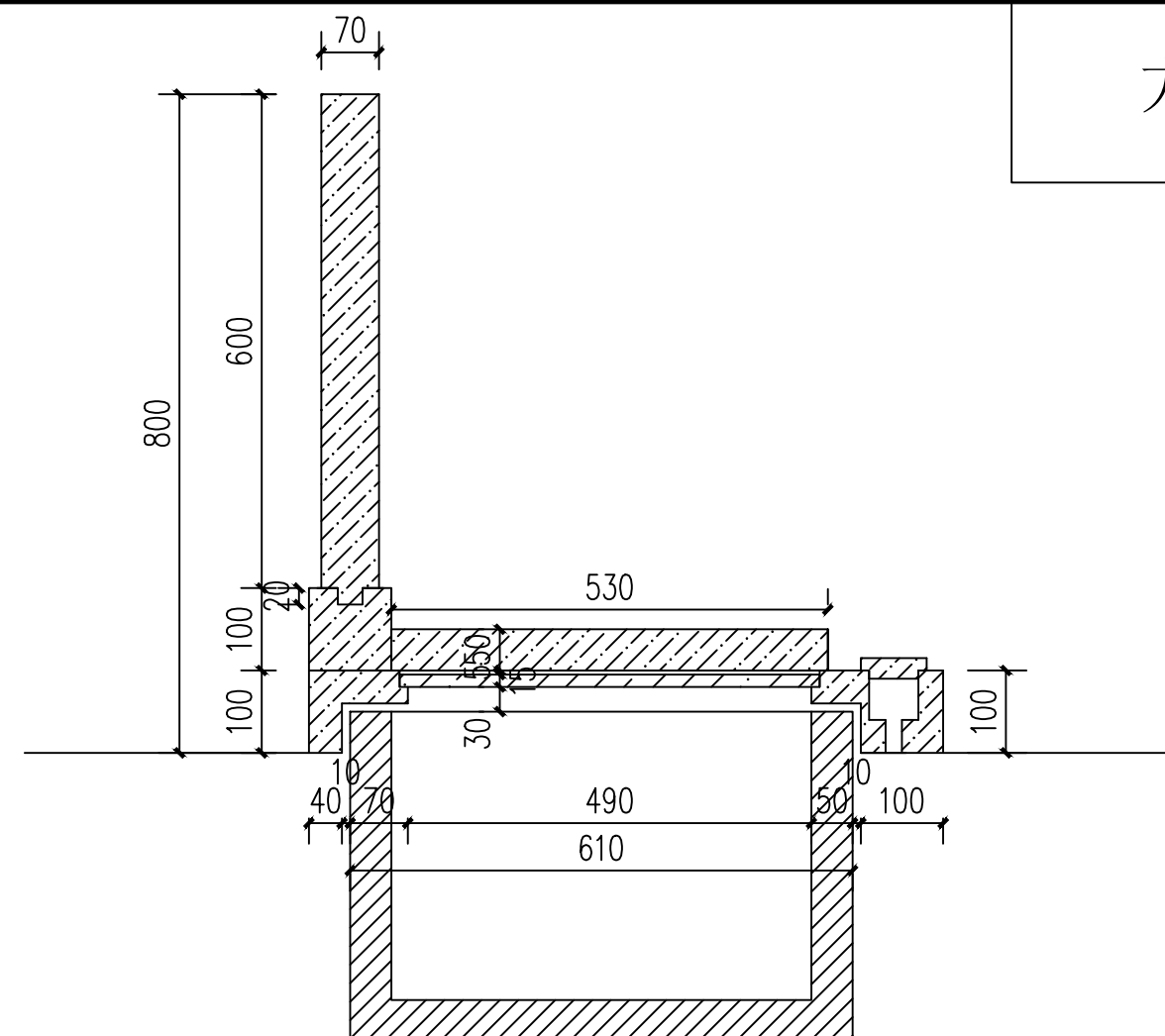
剖面图
